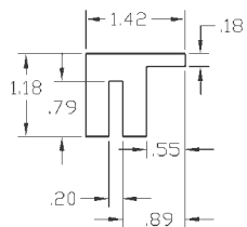
UHMW: 3201124 OF/UHMW: 3203124
